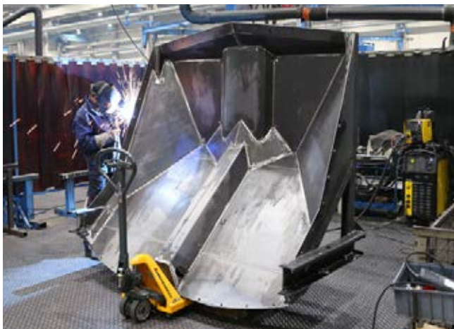
W zakładzie ZOELLER TECH w Rekowiu Górnym główne elementy każdej śmieciarki, tj. skrzynia ładunkowa, płyta wypychająca i odwłok są spawane na trzech osobnych liniach, po czym trafiają do komory śrutowniczej.
